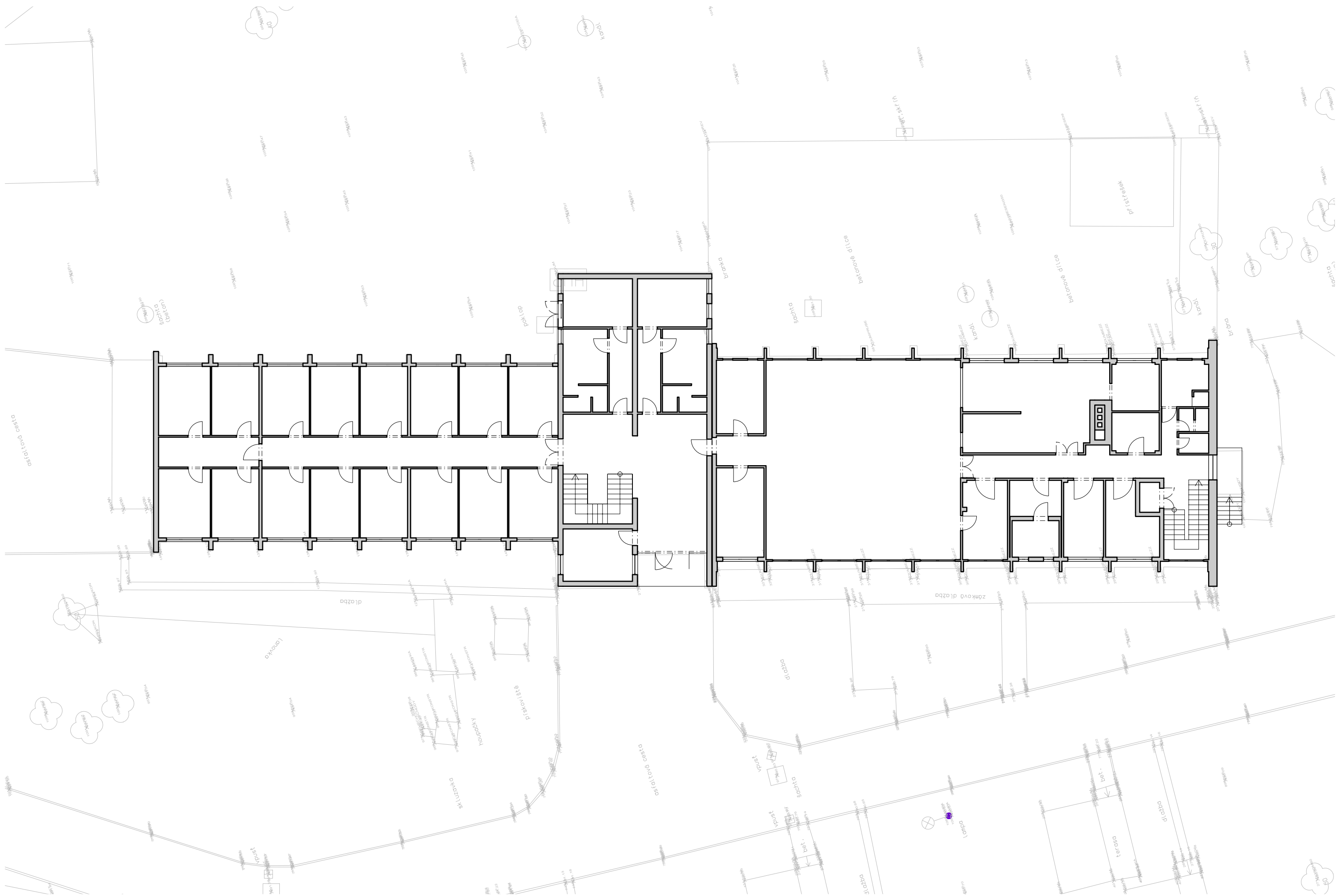
stávající stav hlavní budovy - půdorys 2.NP
