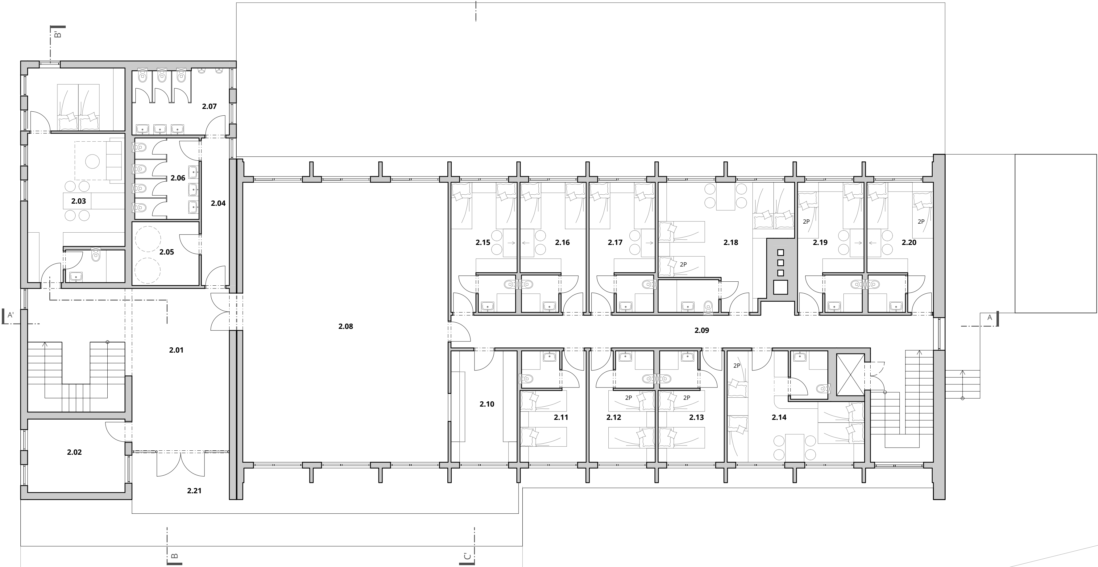
návrh hlavní budovy - půdorys 2.NP
