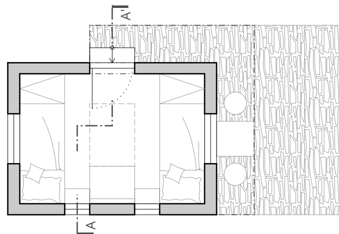
půdorys - varianta s přistýlkou
