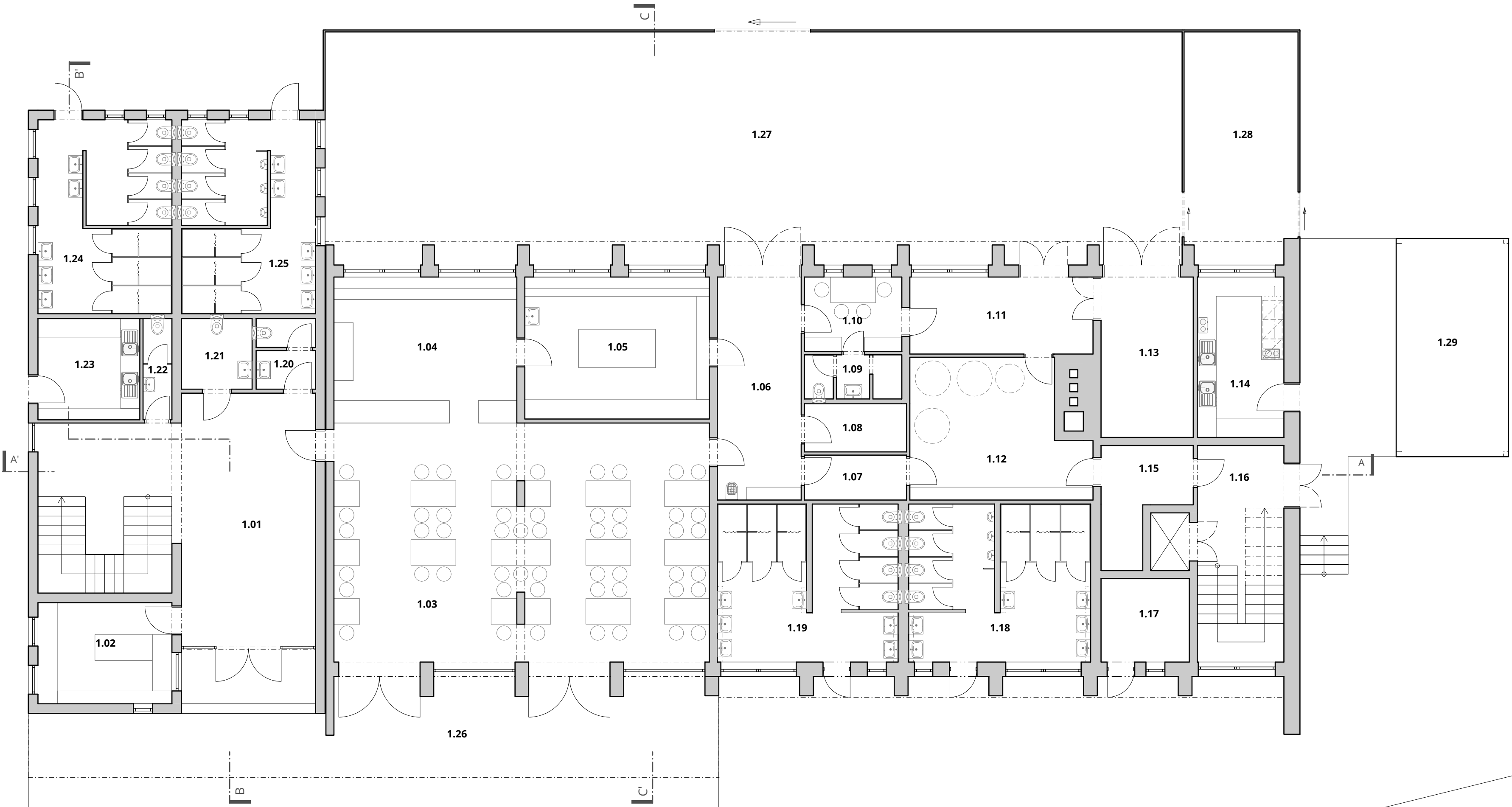
návrh hlavní budovy - půdorys 1.NP
