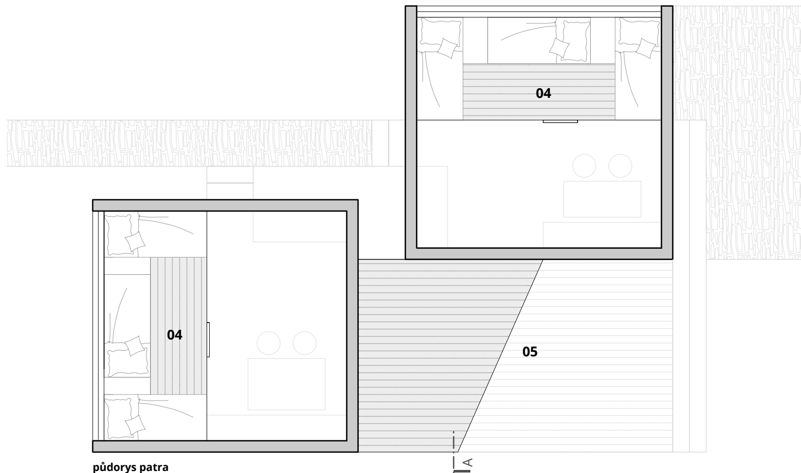
chatka 01 - půdorysy a řez
