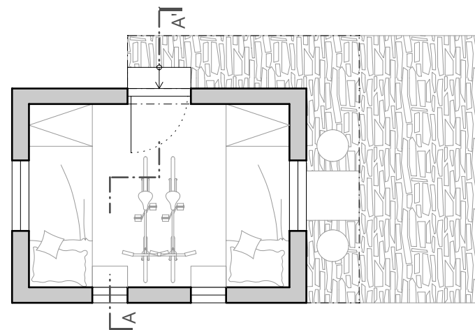
půdorys - varianta s koly
