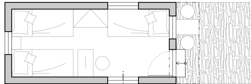
půdorys - varianta s přístýlkou
