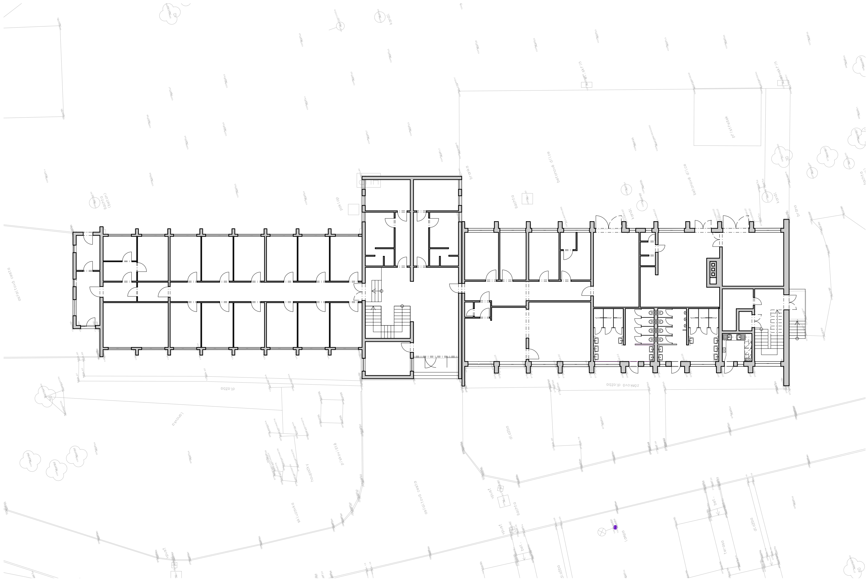
stávající stav hlavní budovy - půdorys 1.NP
