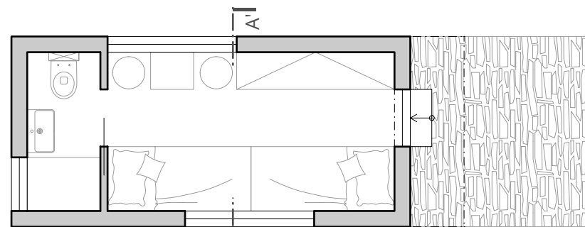
půdorys - varianta se zázemím
