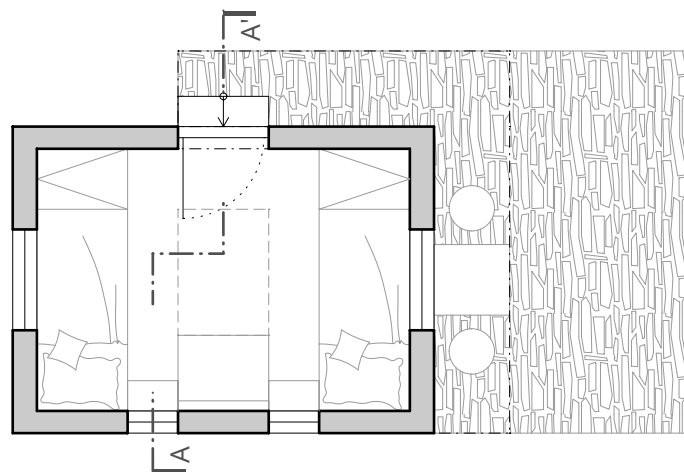
půdorys - varianta s přístýlkou
