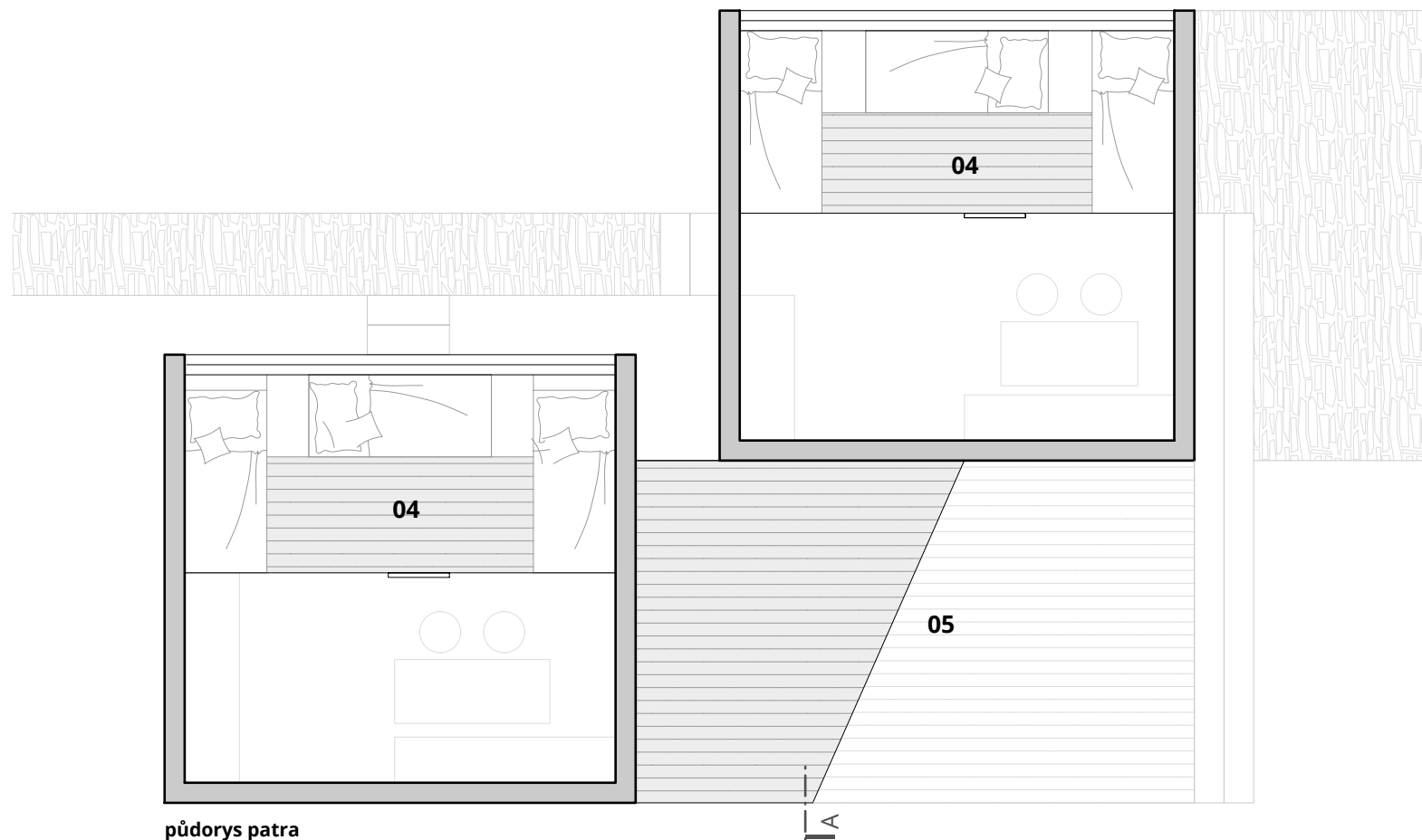
chatka 02 - půdorysy a řez
