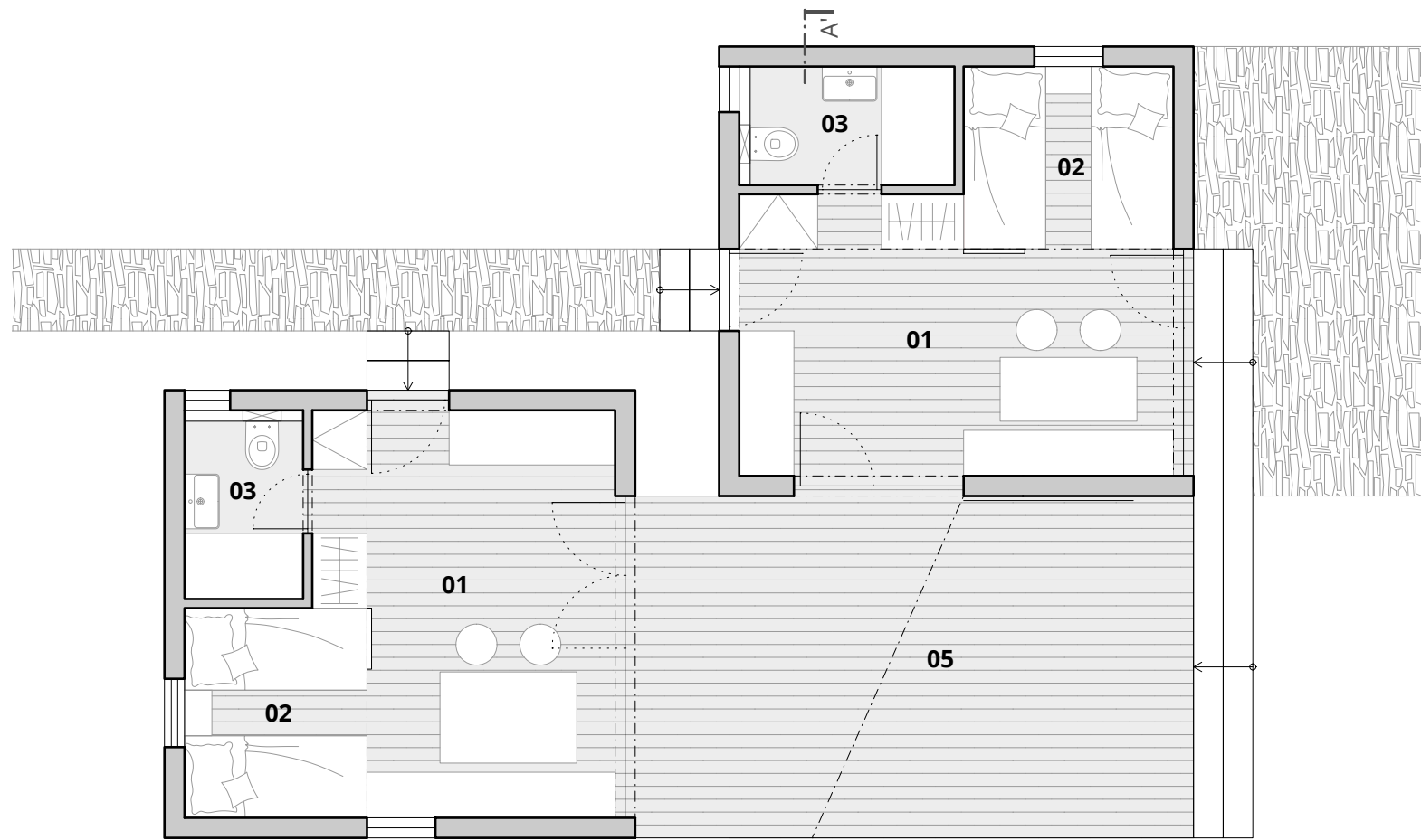
půdorys 1.NP
